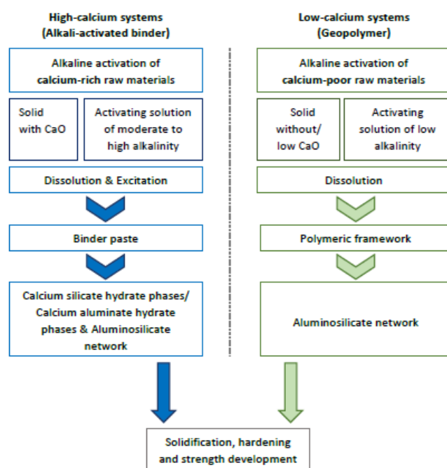
Figuur 2: Schematische weergave reactiemechanisme calcium-rijke en calcium-arme bindmiddelen
